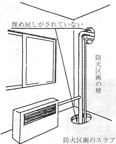
防火区画のスラブ 〔埋め戻しがされていない貫通部〕
